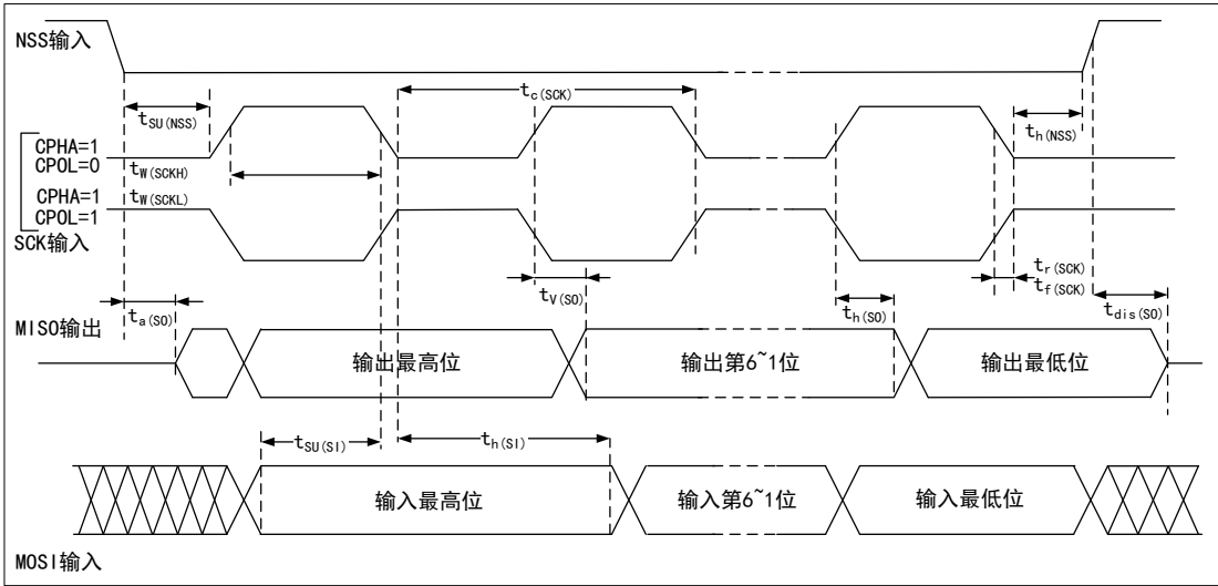
图9 SPI 时序图—从模式和 CPHA=1
