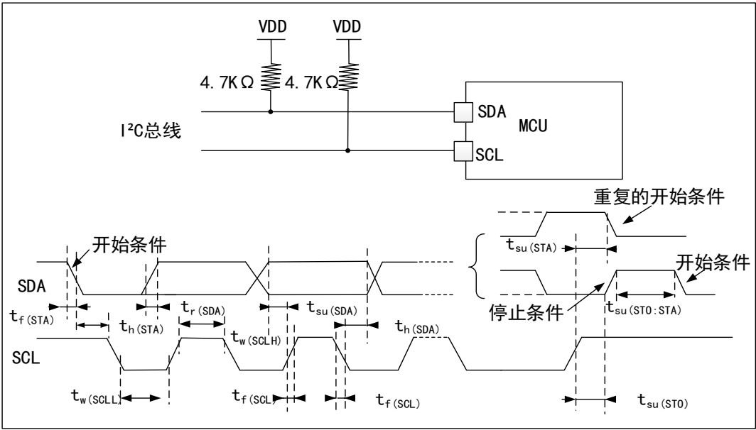
图7 总线交流波形和测试电路
