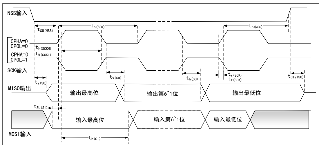
图8 SPI 时序图—从模式和 CPHA=0
