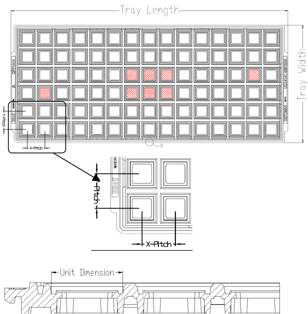
图13 纸盘尺寸
