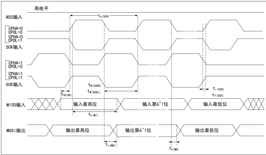
图10 SPI 时序图—主模式
